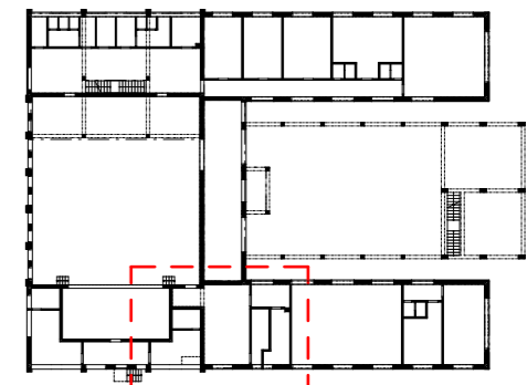
SCHÉMA OBJEKTU
